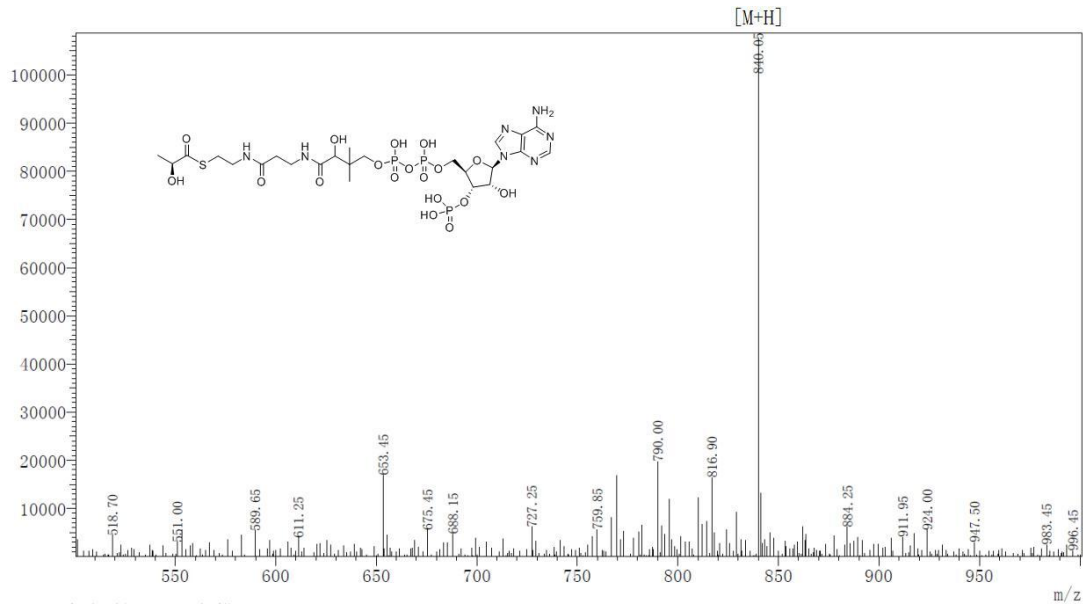
质谱
