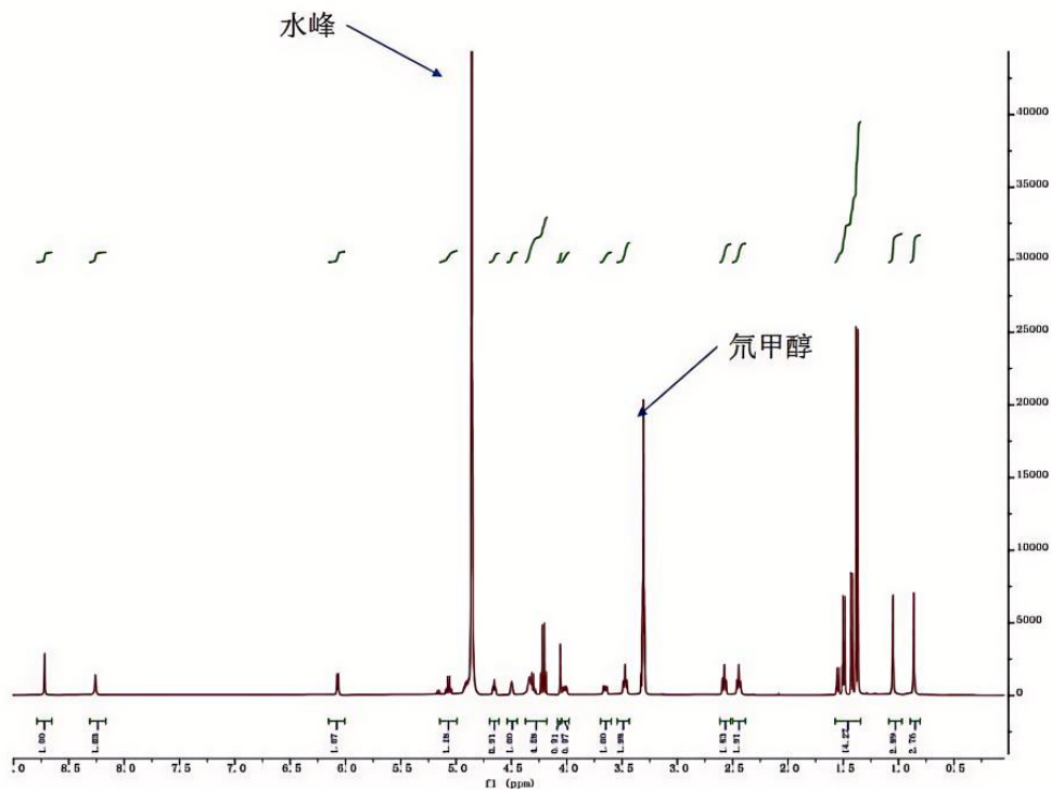
氢谱
